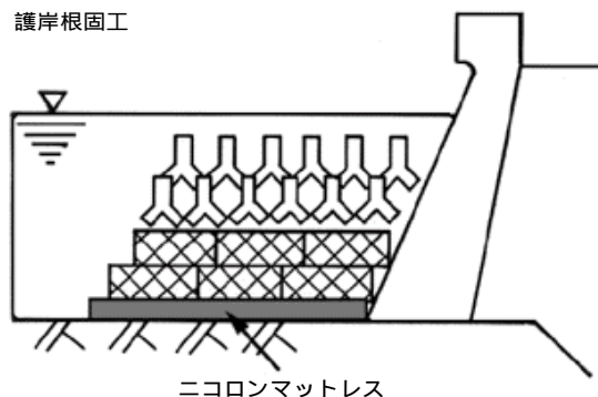
護岸根固工
